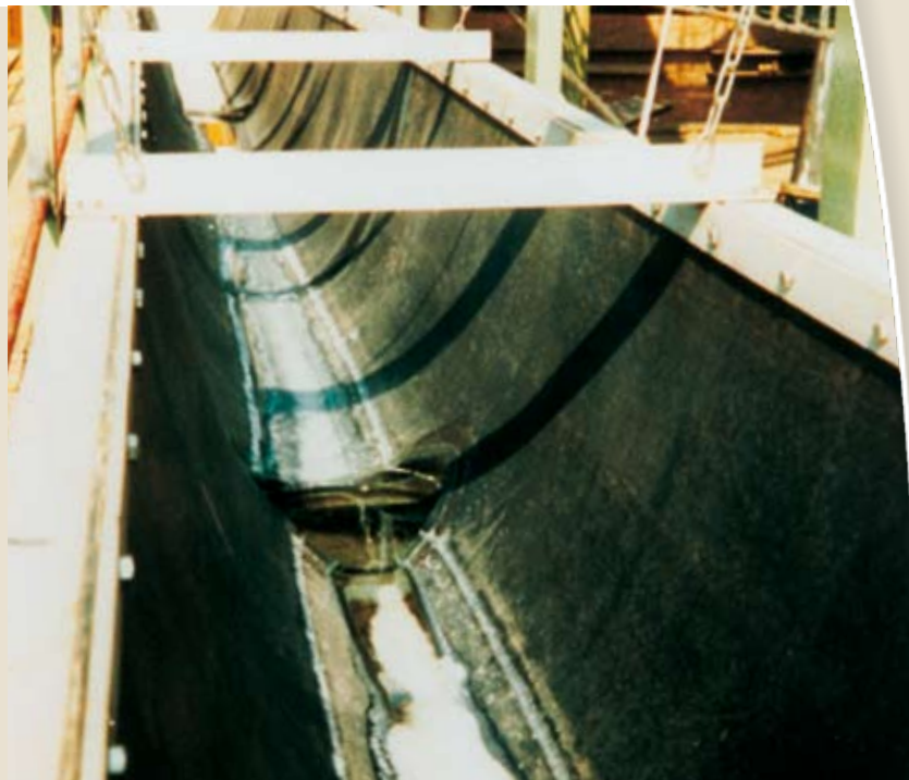
футеровка желобов
